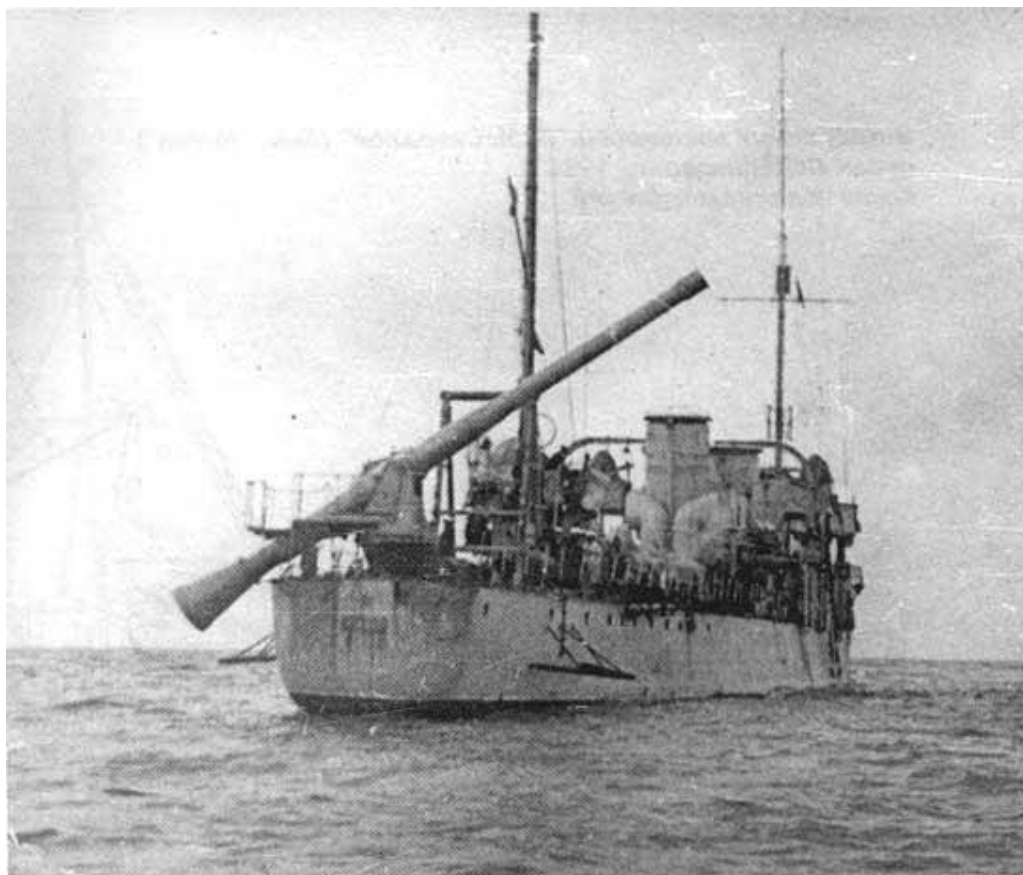
Destructor ruso con cañón sin retroceso de 305 mm
